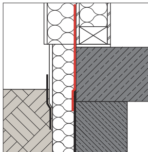
Sokkelfafdichting bij houtskeletbouw
