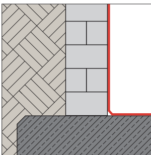
Curatieve afdichting binnen
