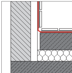
Afdichting onder tegels en plavuizen
