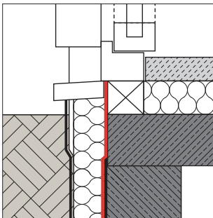
Afdichting bij kozijnen op maaiveldhoogte
