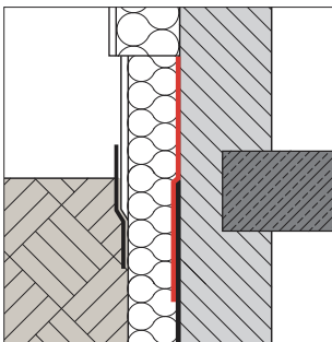
Sokkelfafdichting
