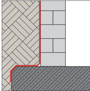
Buitenafdeling beneden maaiveld
