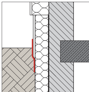
Stucafdichting
