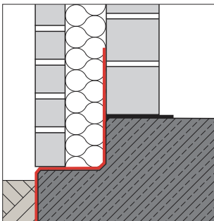
Funderingsafdichting bij spouwmuren
