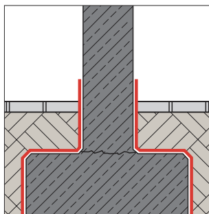
Afdichting van funderingen en kolommen
