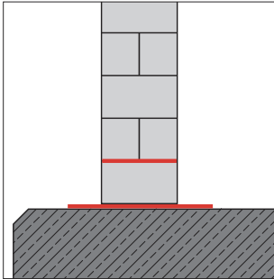
Afdichting in en onder opgaande muren
