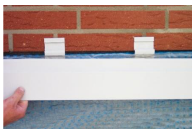
Abb. 4 Anbringen der DS Protect AL. Leiste einfach in DS Protect Clips einrasten lassen.
