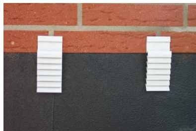
Abb. 1 DS Protect Clips im Abstand von ca. 25 cm verübeln.
