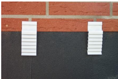
Abb. 1 DS Protect Clips [basic] im Abstand von ca. 25 cm verdübeln.
